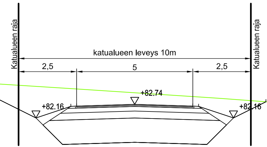
LEIKKAUS PL40
