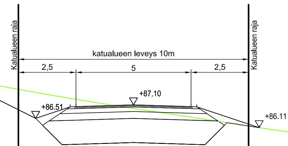
LEIKKAUS PL 140
